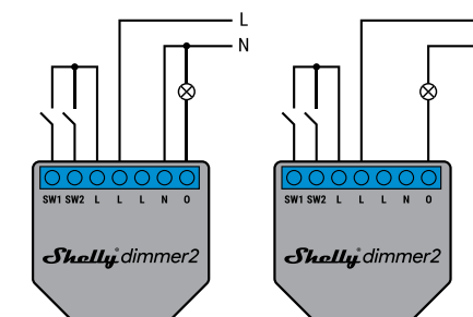
Стандартно окабеляване с неутрала
