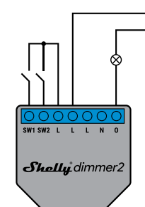
Няма неутрално окабеляване
