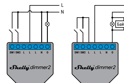
Стандартно окабеляване с нула и SW, свързани към нулата
