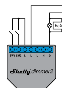
Без нулево окабеляване и без изисквания за минимален товар
